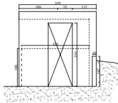
既有廁所北向立面圖
